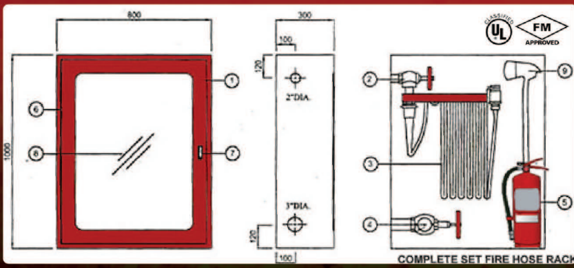
ទូរដាក់ឧបករណ៍ពន្លត់អគ្គិភ័យ
