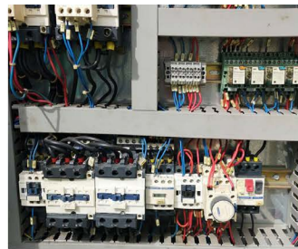
Tower Crane Terex comedil ម៉ាក CTT 91-5
